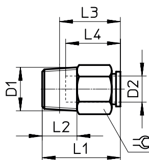
Rosca R
