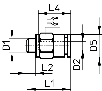
Rosca M
